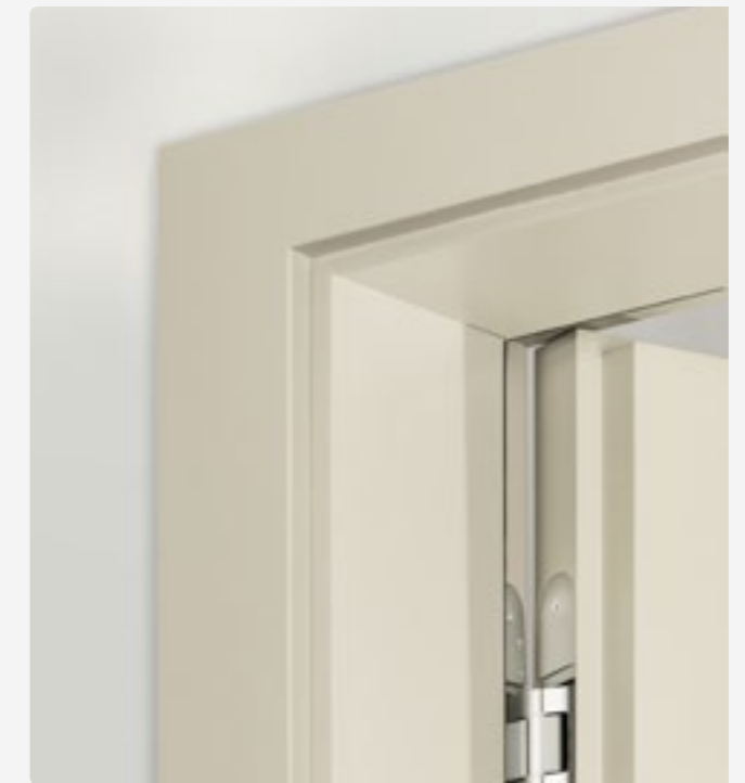
Die neue Zarge überdeckt jeweils den Wandansatz mit der Bekleidung. Das macht Tapezieren oder aufwändiges Nacharbeiten überflüssig.
