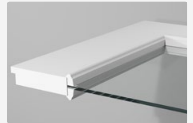
Türblatt mit Lichtausschnitt, Glasleiste Typ B
