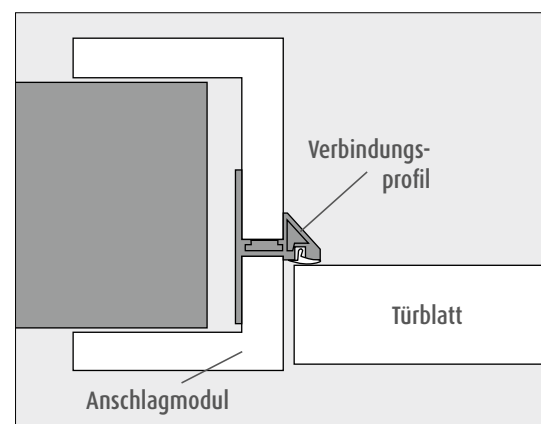
Querschnitt Modell HGM Premium PUR
